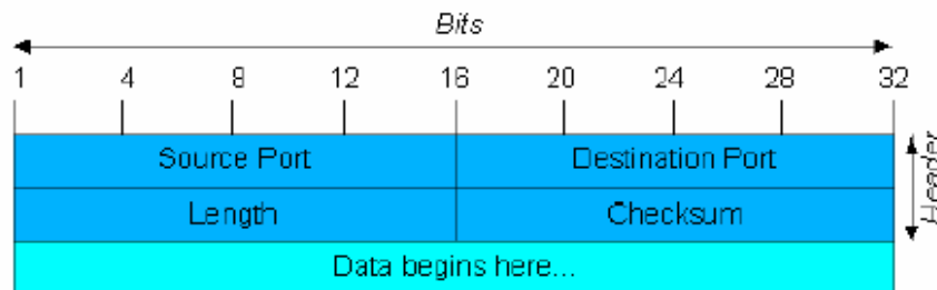
UDP Datagram
